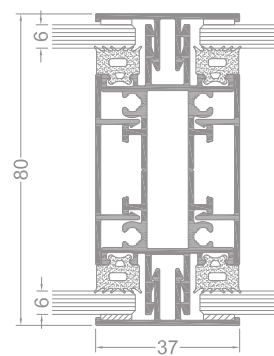
przekrój przez OFFICE (OF002+OF001+OF003)
